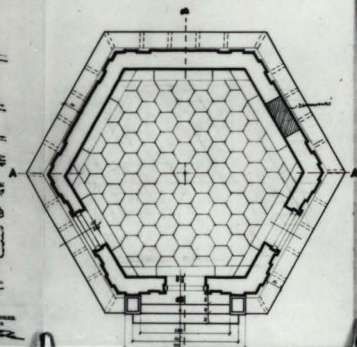
RZUT POZIOMY 1:50
