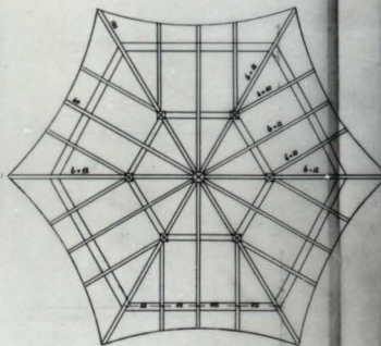
RZUT WIEŻBY DACHOWEJ 1:50
