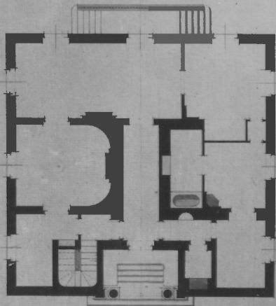
Plan du Rez-de-chaussée de l'Héritage à Lozintzé
