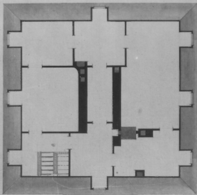
Plan du Rez-de-chaussée de l'Héritage à Lozintzé
